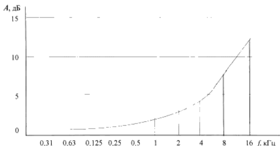
Рисунок 5.2 — АЧХ цепи предуслаживания с постоянной времени 50 мс
