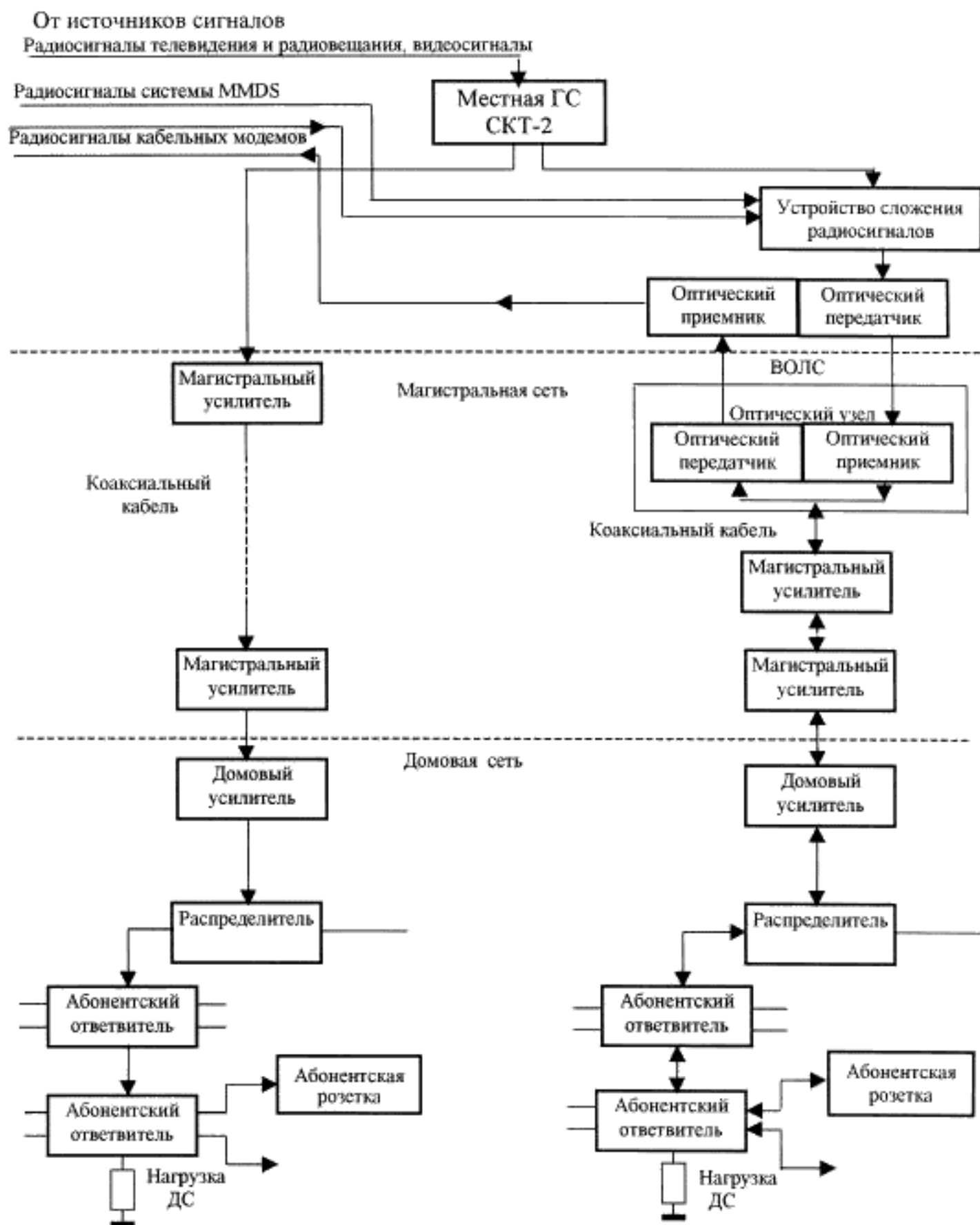
Рисунок 4.2 — Структурные схемы районной кабельной распределительной сети СКТ-2
