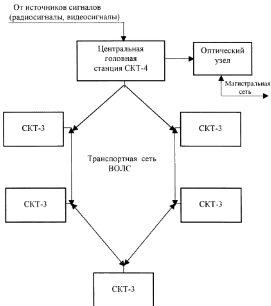
Рисунок 4.4 — Структурная схема региональной кабельной распределительной сети СКТ-4
