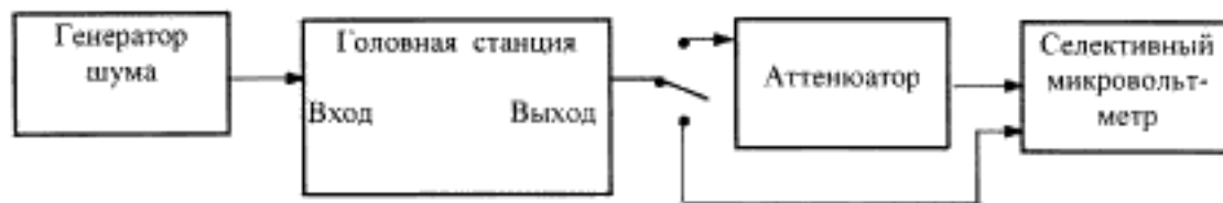
Рисунок 7.10 — Структурная схема для измерения коэффициента шума
