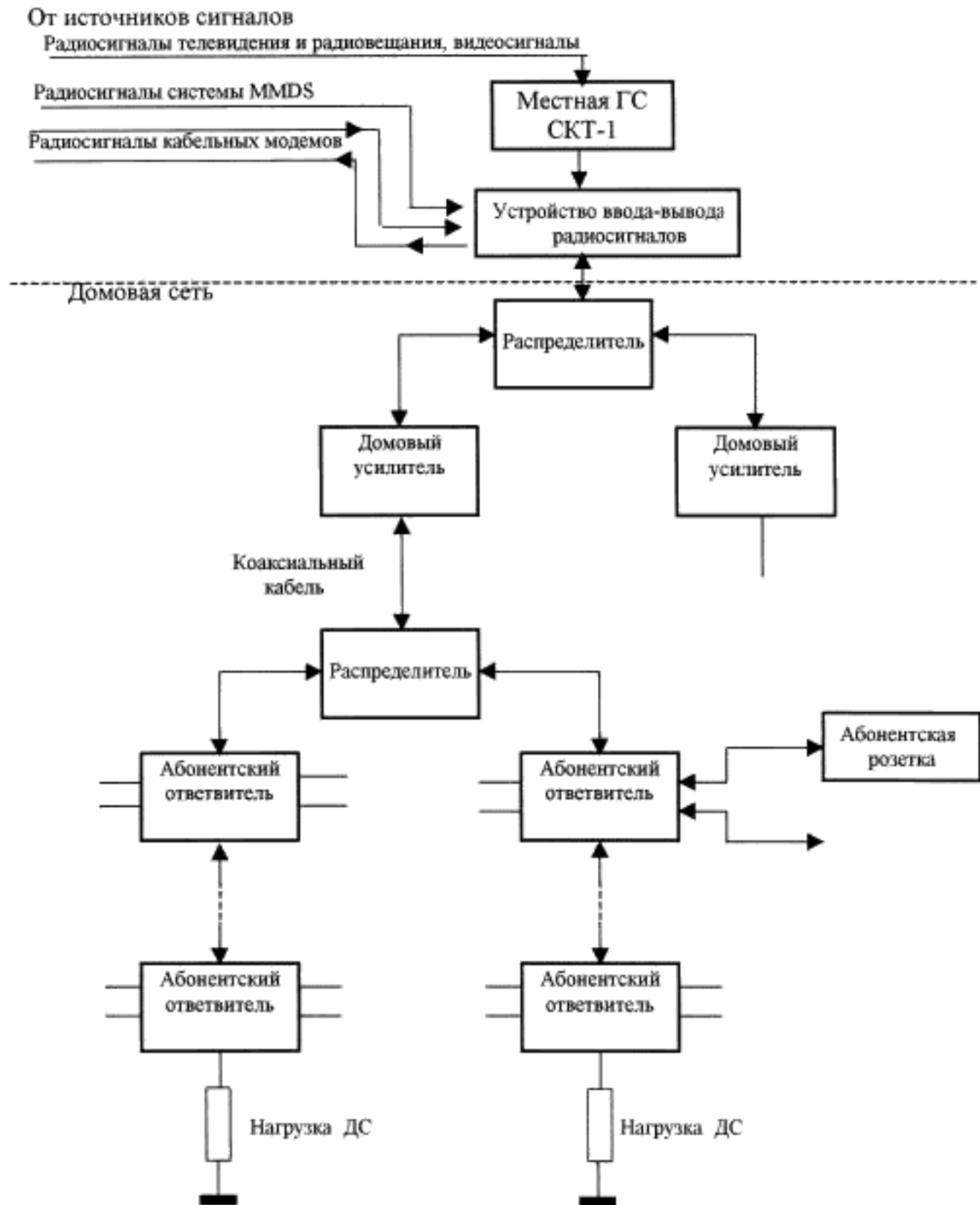
Рисунок 4.1 — Структурная схема местной кабельной распределительной сети СКТ-1
