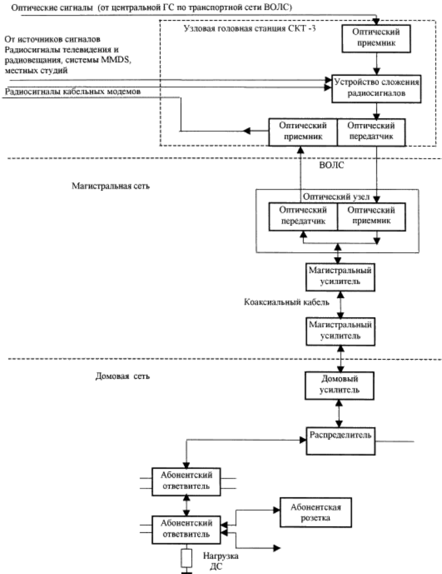
Рисунок 4.3 — Структурная схема городской кабельной распределительной сети СКТ-3
